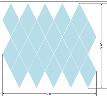
арт.: Серебро ромб 57 Цена за матрицу - 17,8 руб Чип: 98x57x4 мм Матрица: 319x348 мм
