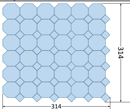
арт.: Серебро КШ Цена за матрицу - 18 руб Чип: 20*20x4 мм Чип: 50*50x4 мм Матрица: 314 мм * 314 мм
